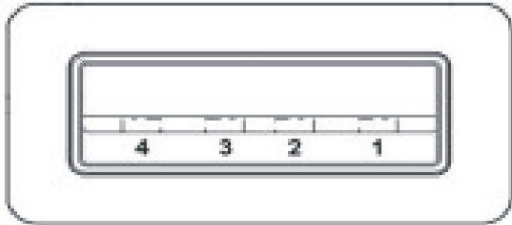
USB-A USB
