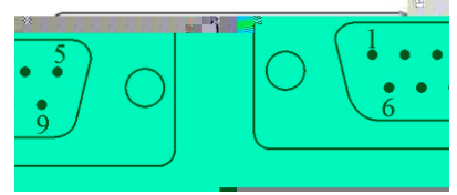
DB9针型
