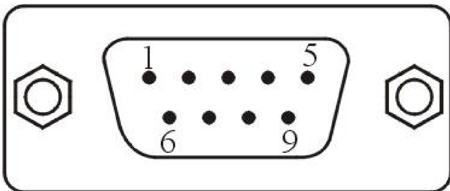
DB9 PIN
