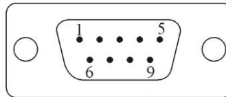
DB9针型
