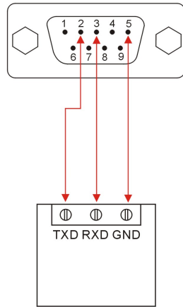
RS-232設備
