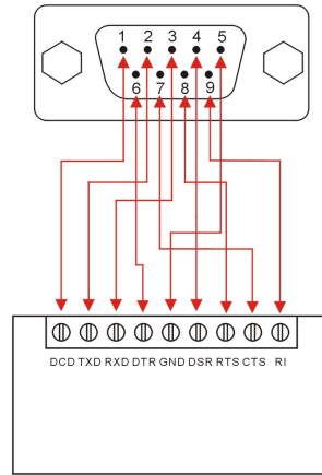
RS-232設備
